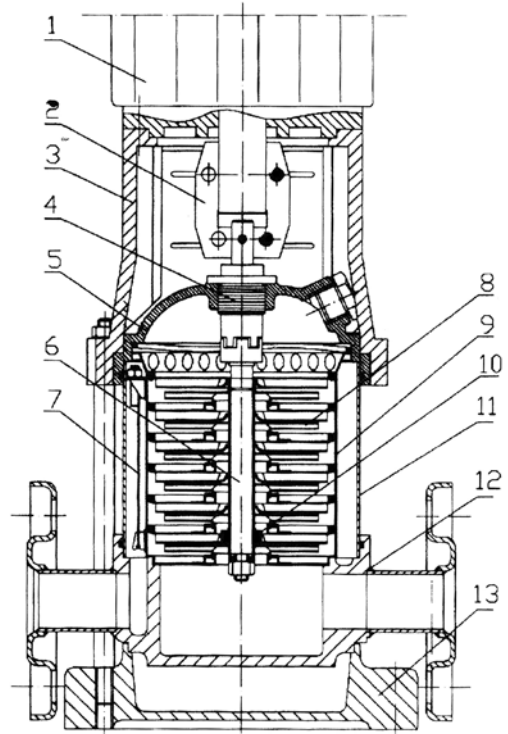
25GDLF2 - 32GDLF5
